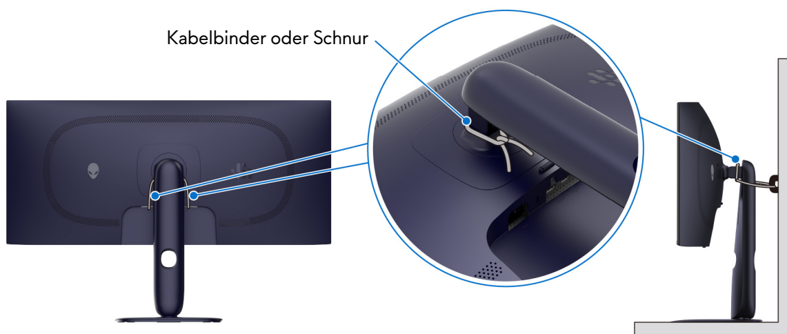
Abbildung 24. Befestigen Sie den Ständerarm an einer Wand, damit der Monitor nicht umfallen kann
