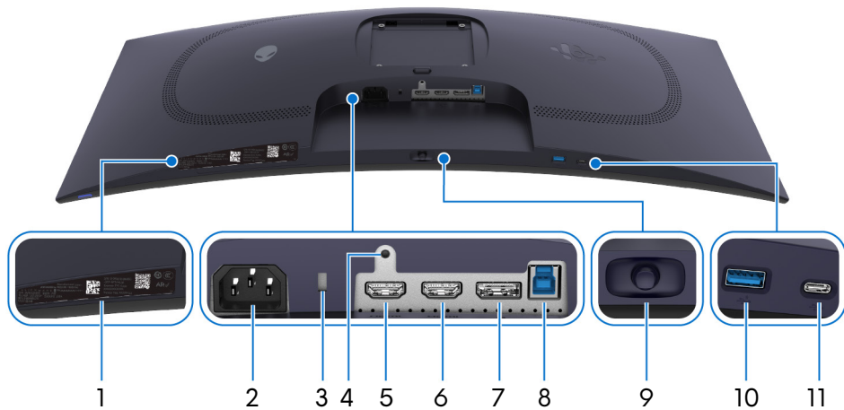
Abbildung 3. Ansicht der Unterseite des Monitors (ohne Monitorständer)
